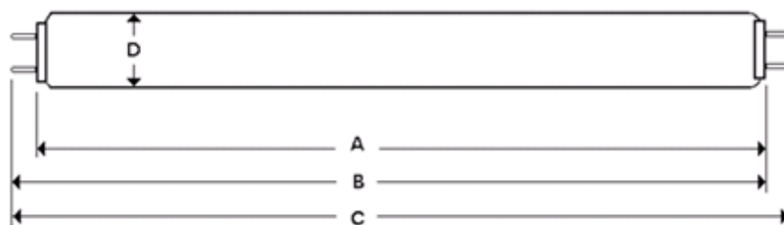
Figura B1: Dimensiones de la lámpara con casquillo G13 y G5
