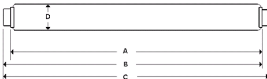
Figura B3: Dimensiones de la lámpara con casquillo R17d
