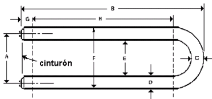
Figura B4: Dimensiones de la lámpara en forma de U
